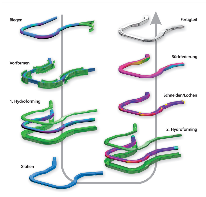
Bild 2: AutoForm Hydro ermöglicht dem Anwender ein vollständiges, virtuelles Tryout von IHU-Prozessen inklusive aller Prozessschritte durchzuführen: Biegen, Vorformen, Innenhochdruckumformen, Glühen, Kalibrieren, Schneiden und Rückfedern (Werkbilder: AutoForm Engineering GmbH, CH-Wilen b. Wollerau, Schweiz)
